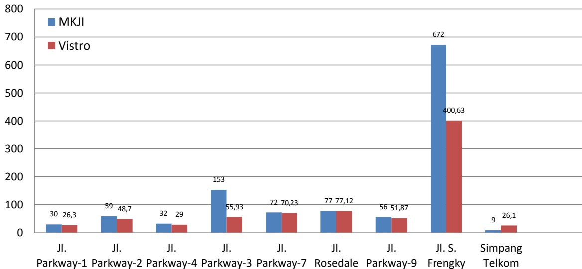
Gambar 8. Perbandingan Nilai D (Perhitungan Vistro dan MKJI)
