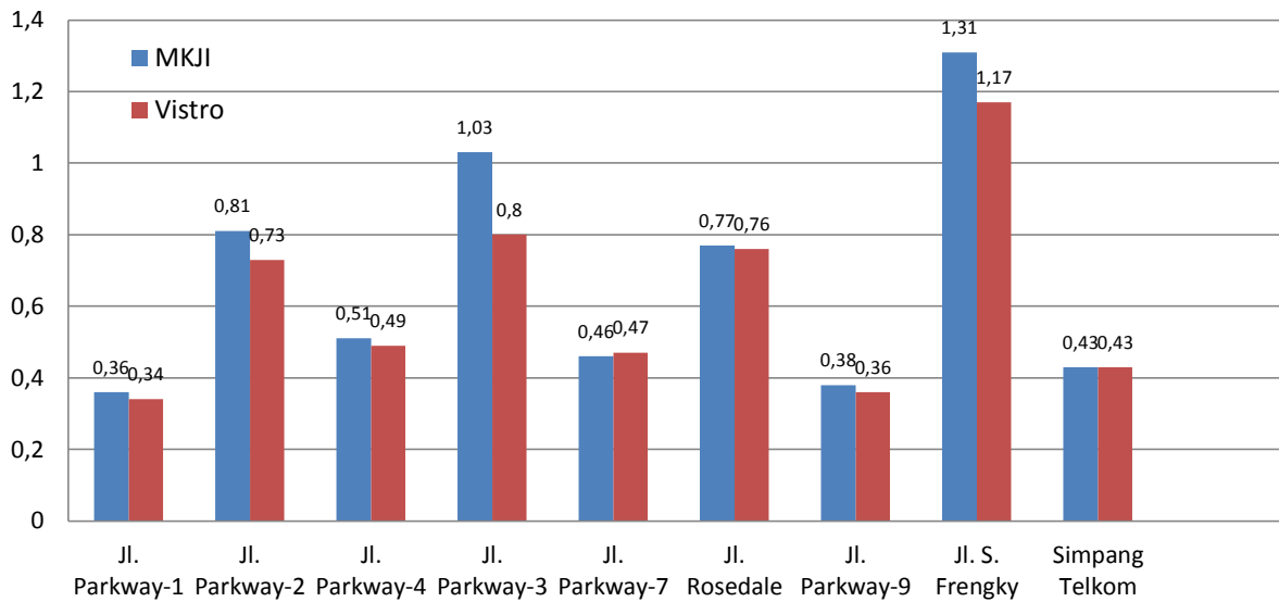
Gambar 7. Perbandingan Nilai DS (Perhitungan Vistro dan MKJI)
