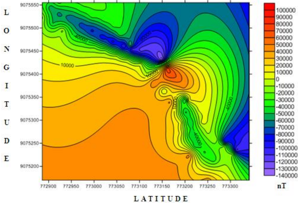
Gambar 5. Pola Kontur hasil Kontinuitas Atas dengan 90 mdatum
