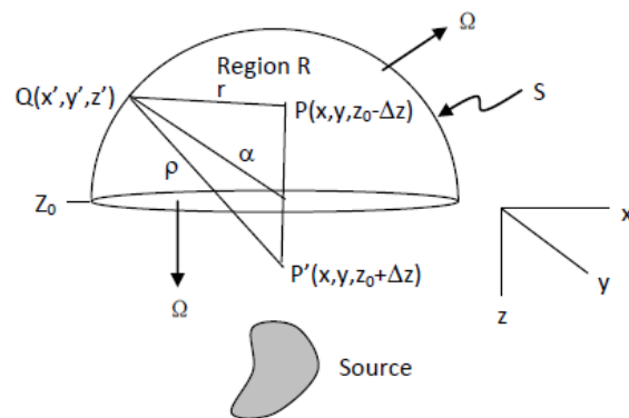
Gambar. 1. Kontinuasi ke atas dari permukaan horizontal (Blakey, 1995)
