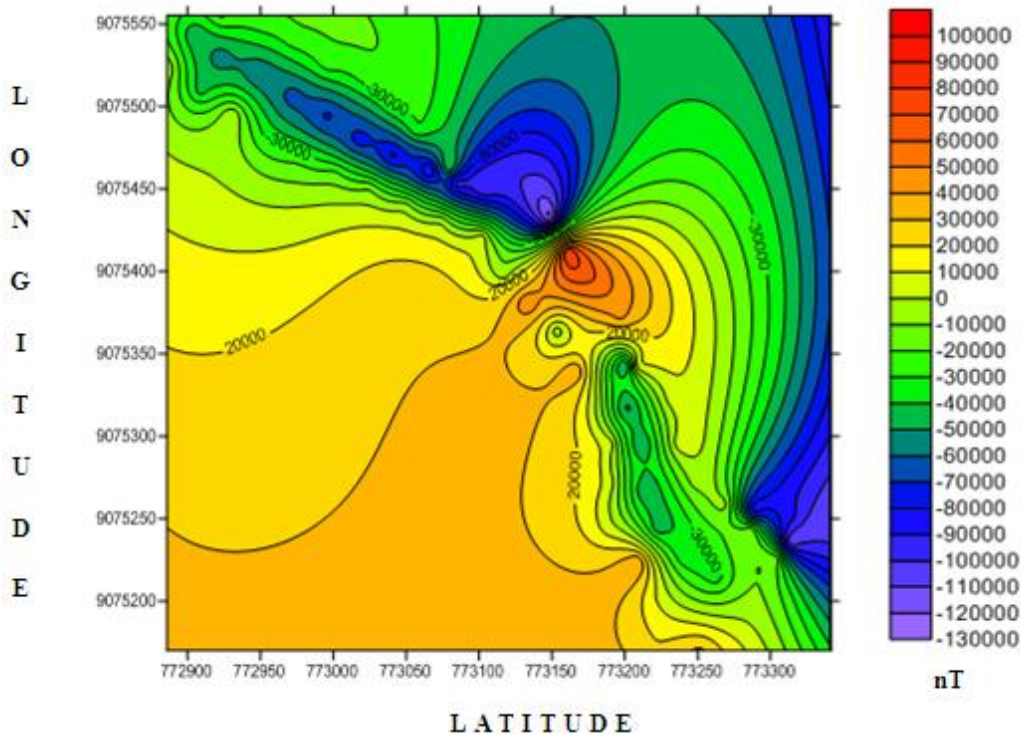
Gambar 3. Pola Kontur hasil Kontinuitas Atas dengan 70 mdatum
