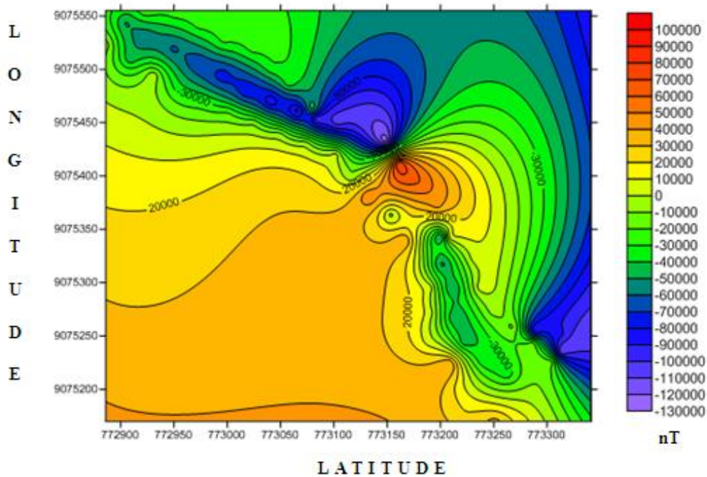
Gambar 4. Pola Kontur hasil Kontinuitas Atas dengan 80 mdatum
