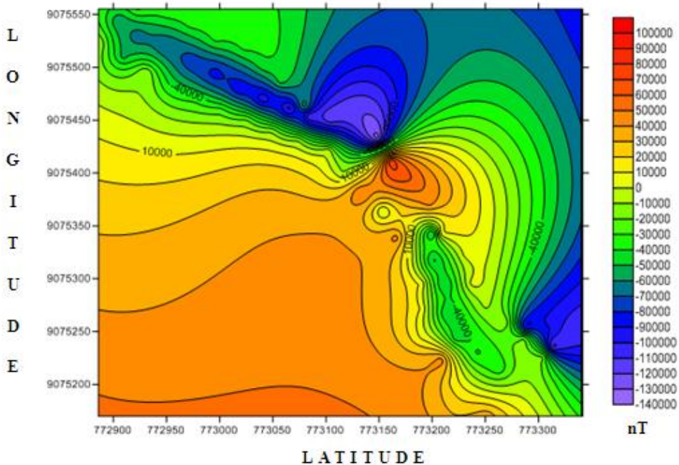
Gambar 6. Pola Kontur hasil Kontinuitas Atas dengan 100 mdatum
