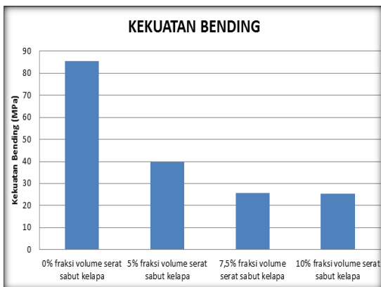
Gambar 1. Grafik Kekuatan Bending pada variasi fraksi serat sabut kelapa
