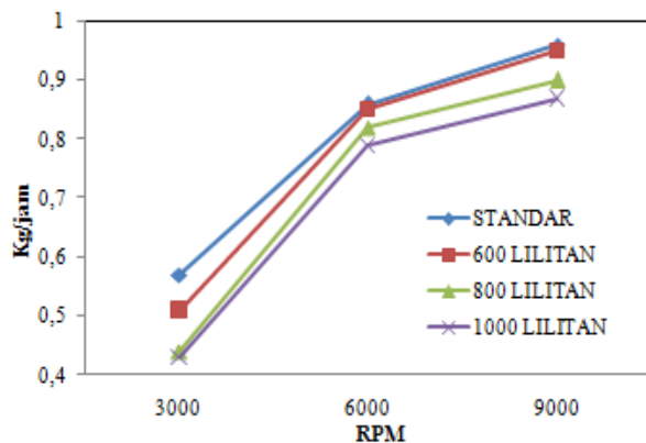
Gambar 7. Grafik perbandingan FC dengan putaran mesin dengan keadaan standar dan menggunakan variasi jumlah lilitan elektromagnet 600 lilitan, 800 lilitan, 1000 lilitan.
