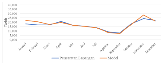
Gambar 6 Grafik Debit Model dengan Debit Bendung Sesudah Kalibrasi Tahun 2017
