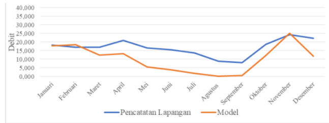
Gambar 3 Grafik Debit Model dengan Debit Bendung Sebelum Kalibrasi Tahun 2017
