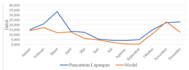
Gambar 2 Grafik Debit Model dengan Debit Bendung Sebelum Kalibrasi Tahun 2013
