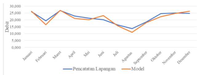
Gambar 7 Perbandingan Grafik Debit Model dengan Debit Bendung Sesudah Kalibrasi dengan Pemodelan ArcSWAT pada Tahun 2022
