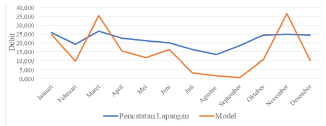
Gambar 4 Grafik Debit Model dengan Debit Bendung Sebelum Kalibrasi Tahun 2022
