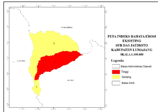
Gambar 9 Pemetaan Indeks Bahaya Erosi Eksisting
