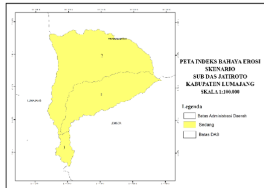
Gambar 11 Peta Indeks Bahaya Erosi Skenario
