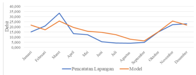
Gambar 5 Grafik Debit Model dengan Debit Bendung Sesudah Kalibrasi Tahun 2013
