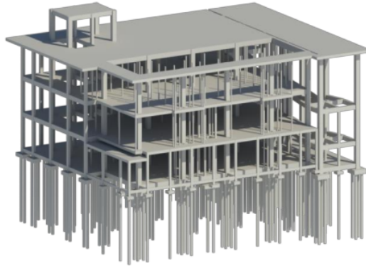
Gambar 2 Pemodelan Revit Sumber : Hasil Pemodelan (2023)
