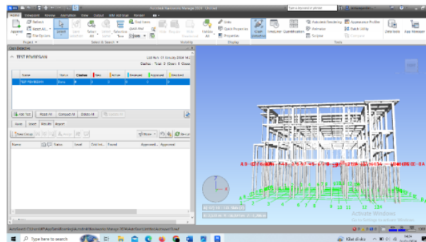
Gambar 3 Clash Detection Sumber : Hasil Pemodelan (2023)
