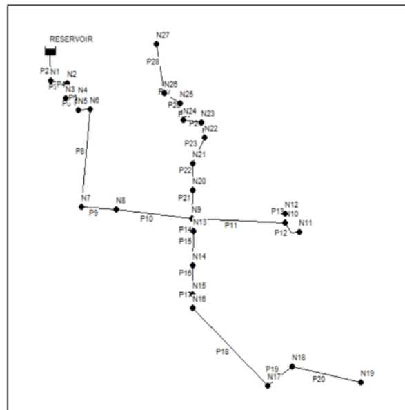
Gambar 1 Penomoran titik dan pipa.
