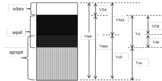
Gambar 1 Skematis Volumetrik Campuran Beton Aspal (Sumber: Sukirman, 2007)
