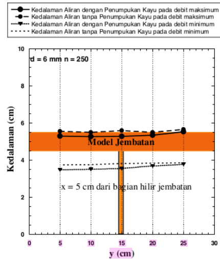
Gambar 13 Kedalaman aliran pada bagian hilir jembatan
