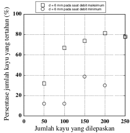
Gambar 8 Persentase jumlah kayu yang tertahan
