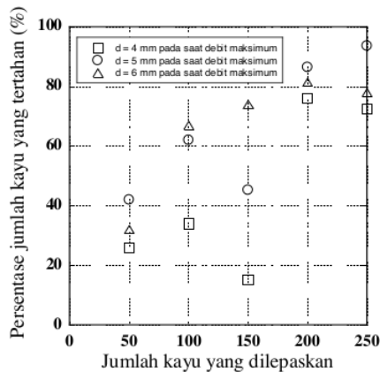
Gambar 9 Persentase jumlah kayu yang tertahan saat debit maksimum
