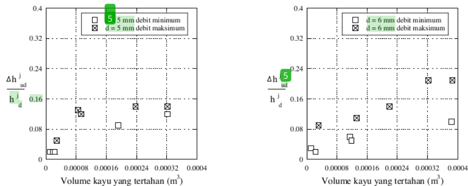
Gambar 16 Hubungan antara backwater rise dengan volume kayu yang tertahan pada model jembatan saat debit aliran mencapai nilai minimum dan maksimum
