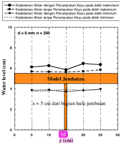
Gambar 12 Kedalaman aliran pada bagian hulu jembatan
