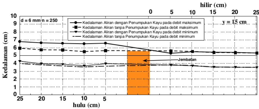
Gambar 14 Kedalaman aliran pada bagian hulu dan hilir model jembatan
