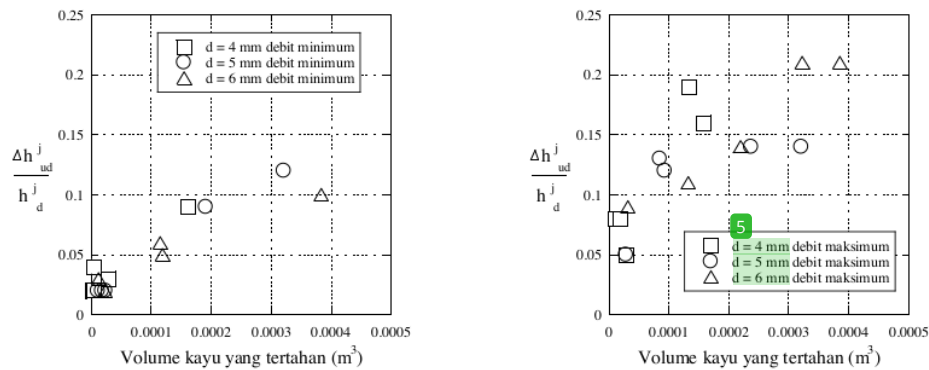
Gambar 15 Hubungan antara backwater rise dengan volume kayu yang tertahan pada model jembatan saat debit aliran mencapai nilai minimum dan maksimum
