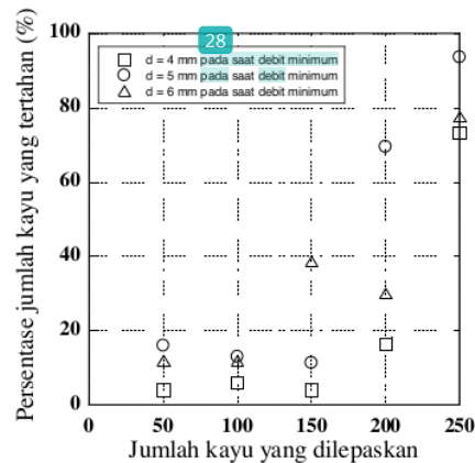
Gambar 10 Persentase jumlah kayu yang tertahan saat debit minimum
