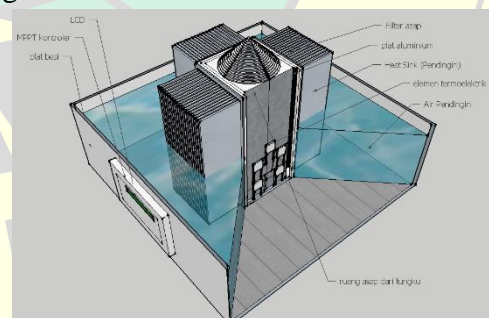
Gambar 4. Desain generator termoelektrik
