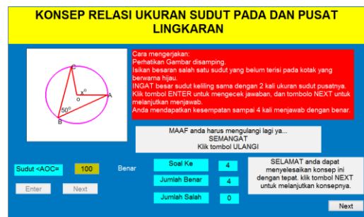
Gambar 7. Relasi Ukuran Sudut Pada lingkaran dan Sudut Pusat Lingkaran
