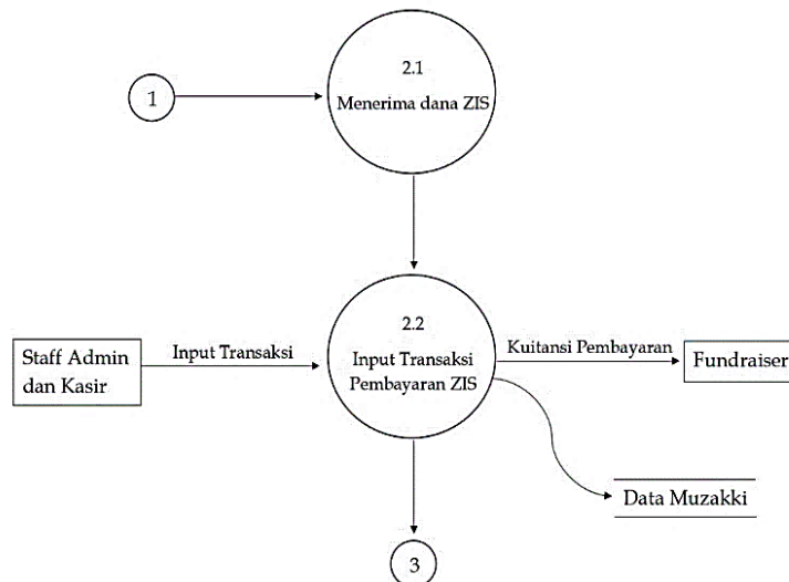
Gambar 4.6. Usulan DFD Penghimpunan Dana ZIS Level 2
