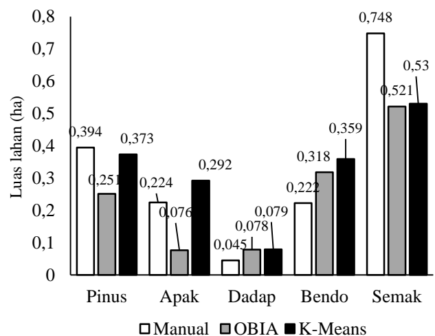
Gambar 7. Luas lahan pada vegetasi tumbuhan berdasarkan perbandingan metode manual (□), OBIA (▒), dan K-Means (■)
