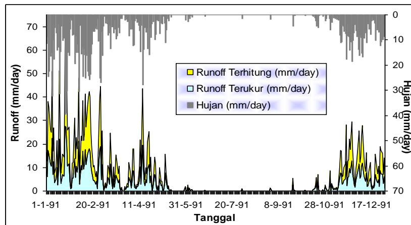
Gambar 13. Grafik runOff terukur dan terhitung hasil kalibrasi DAS Bedadung
