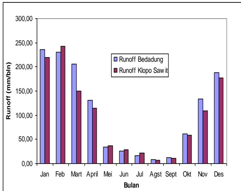
Gambar 4. Grafik rata-rata runoff bulanan DAS Bedadung Dan DAS Klopo Sawit
