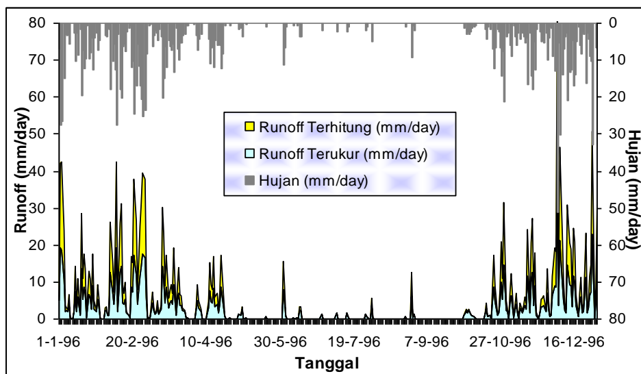
Gambar 10. Grafik runoff terukur dan terhitung hasil Validasi DAS Klopo Sawit
