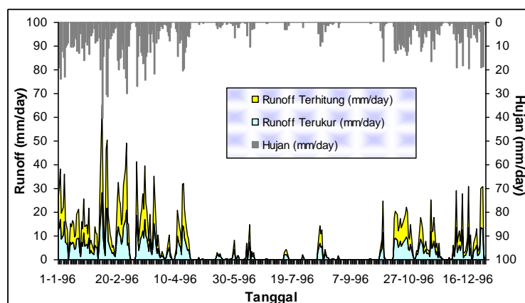
Gambar 15. Grafik runoff terukur dan terhitung hasil validasi DAS Bedadung
