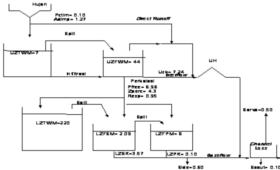
Gambar 8. Struktur model sacramento DAS Klopo Sawit
