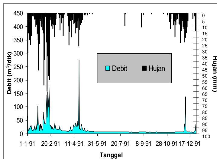
Gambar 6. Grafik analisis data untuk kalibrasi DAS Klopo Sawit
