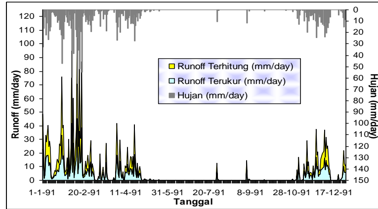
Gambar 7. Grafik RunOff terukur dan terhitung hasil kalibrasi DAS KlopoSawit
