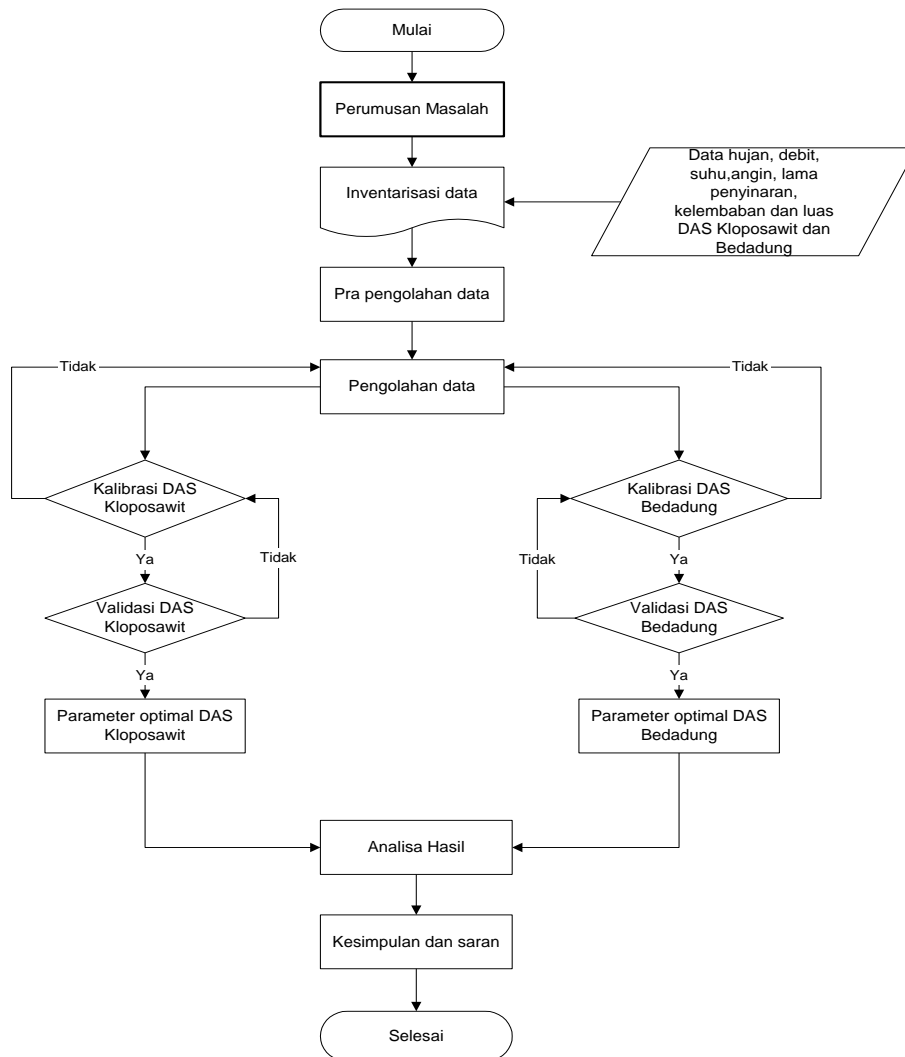
Gambar 2. Diagram alir tahapan penelitian
