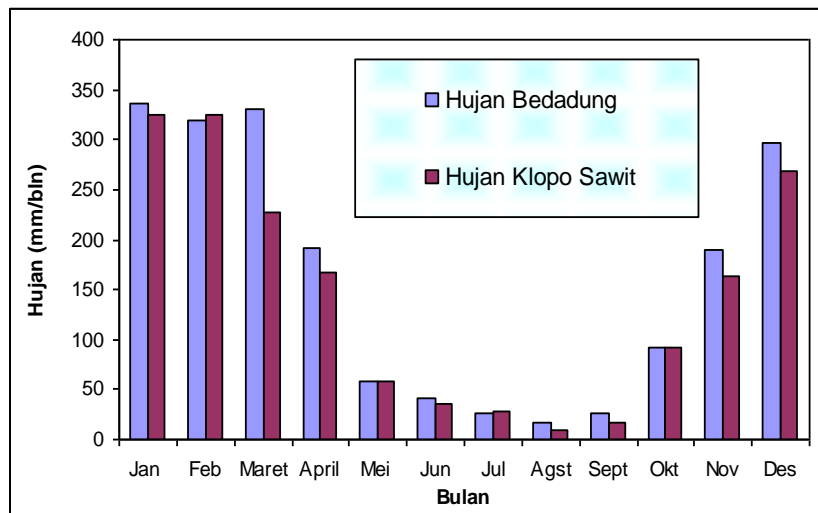
Gambar 3. Grafik perbandingan hujan bulanan DAS Bedadung dan DAS Klop Sawit.
