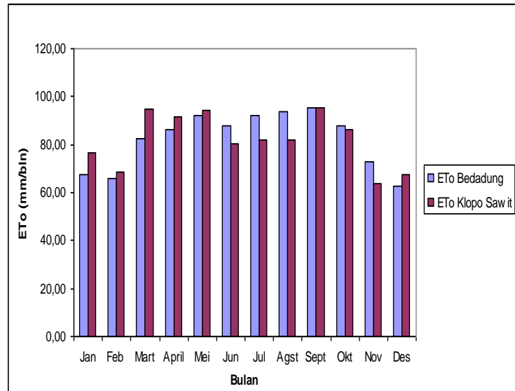
Gambar 5. Grafik evapotranspirasi potensial bulanan DAS Bedadung dan DAS Klopo Sawit
