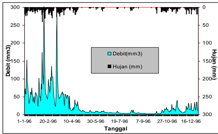
Gambar 12. Grafik analisis data untuk validasi DAS Bedadung
