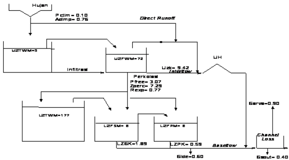
Gambar 14. Struktur model Sacramento DAS Bedadung
