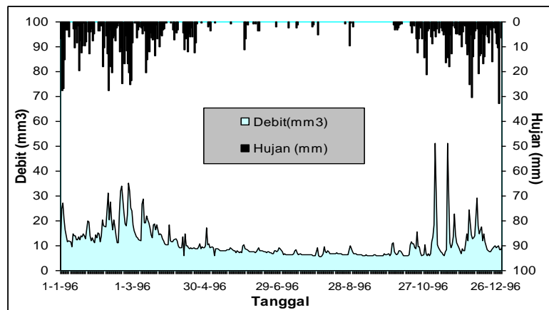
Gambar 9. Grafik analisis data untuk validasi DAS Klopo Sawit
