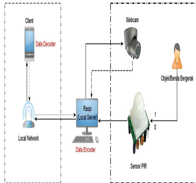
Gbr. 1 Blok diagram
