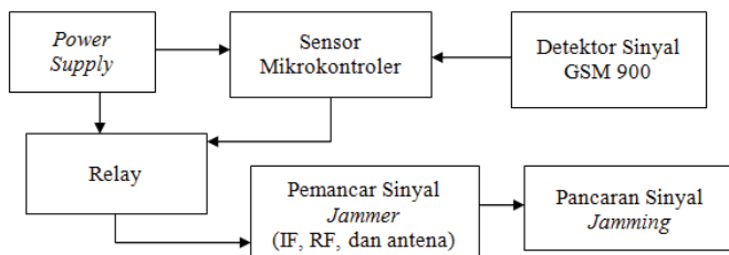
Gambar 2. Diagram Blok Sistem
