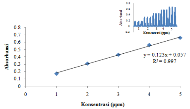
Gambar 6. Kurva larutan standar Fe(II) dengan metode Flow Injection Analysis pada \lambda=510 nm dengan volume 1.10-Fenantrolin maksimum = 0.20 mL dan laju alir = 0.89 mL/min
