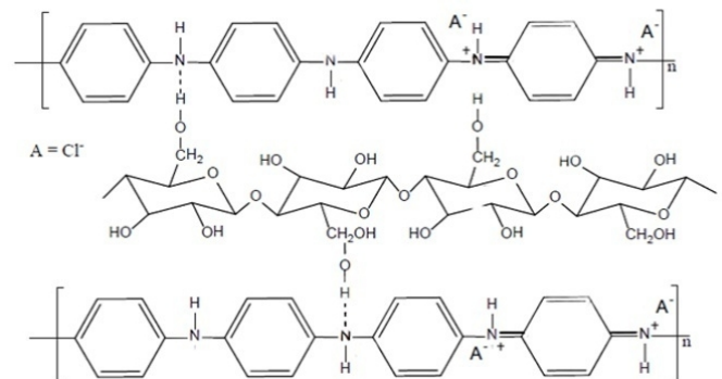
Gambar 4. Struktur Komposit Polianilin-Selulosa Bakteri [14].
