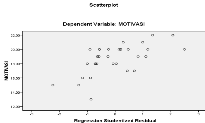
Gambar 2. Uji Heteroskedastisitas
