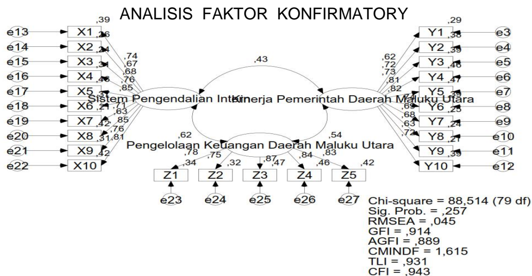
Gambar 2 Uji Validitas dan Reliabilitas dengan Confirmatory Faktor Analysis
