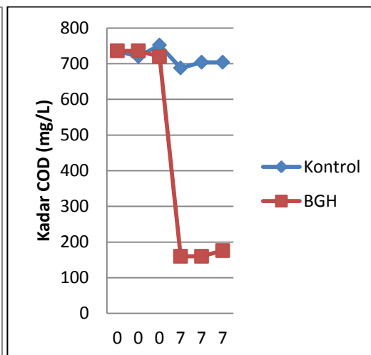
Grafik 3b. Penurunan Kadar COD
